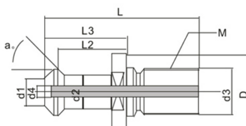
FOR DIN 69872
